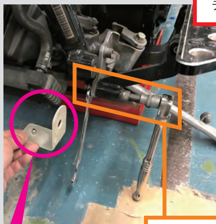
プライマリー側ステー
